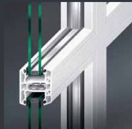
Glasteilende Sprosse
